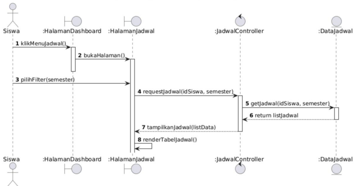
Sequence Diagram - Melihat Jadwal Pelajaran
