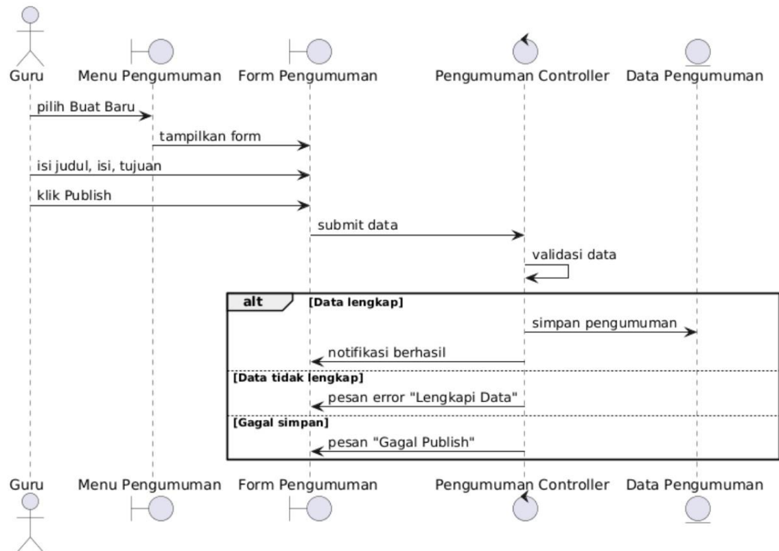
Sequence Diagram - Membuat Pengumuman
