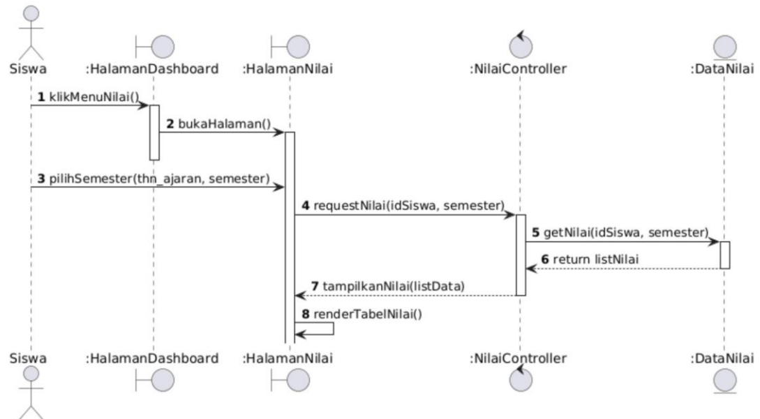
Sequence Diagram - Melihat Nilai
